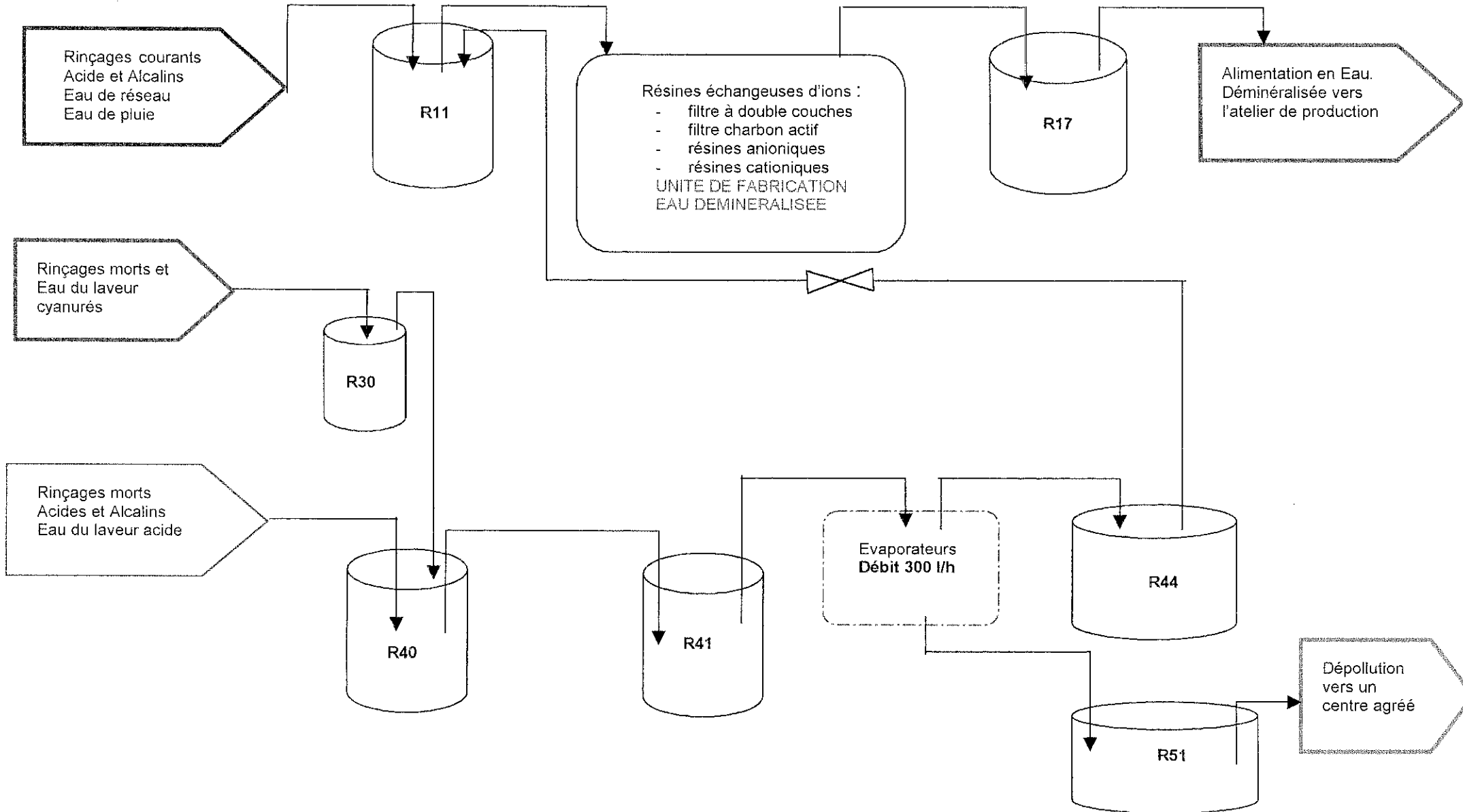
Figure 1: Schéma du procédé de la station de recyclage
